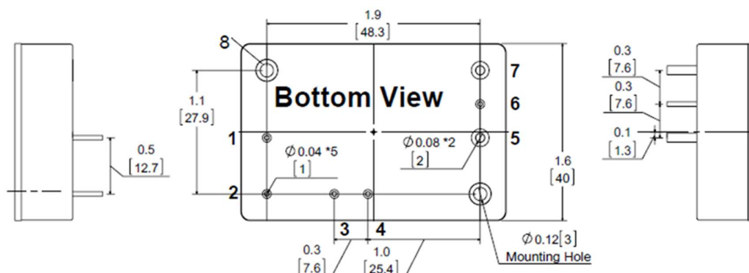
尺寸图
